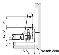
Minimálna svetlá výška zásuvky pre držiak chrbita typu B
