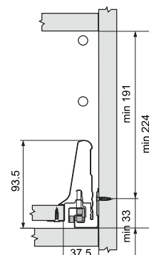
Minimálna svetlá výška zásuvky pre držiak chrbita typu D
