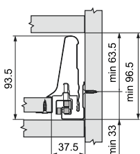
Minimálna svetlá výška zásuvky pre držiak chrbita typu B
