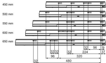
Pozície skrutiek vodiacich lišt s nosnosťou 50 kg
