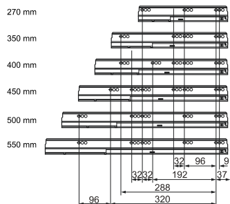
Pozície skrutiek vodiacich lišt s nosnosťou 30 kg
