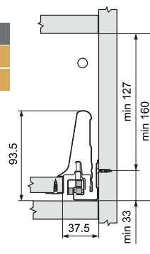
Minimálna svetlá výška zásuvky pre držiak chrbita typu B
